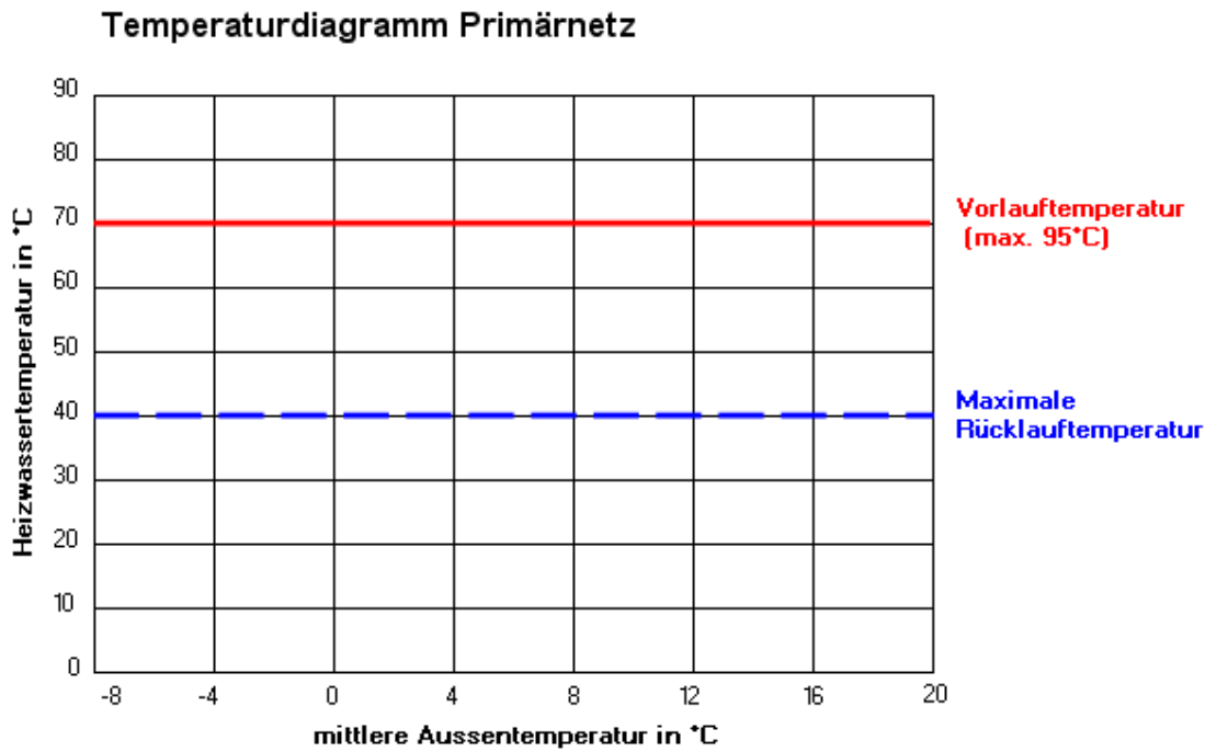
Abbildung 1: Temperaturdiagramm Primärnetz
